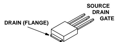
JEDEC TO-251AA
